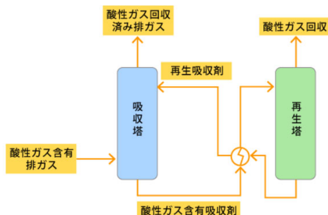
酸性ガス吸収 プロセスフロー（例）
