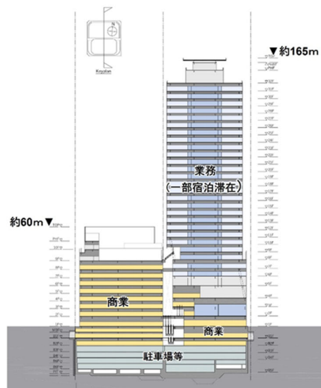
完成予想パース・断面イメージ
