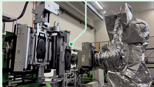
REX-ROBO®による交換作業
